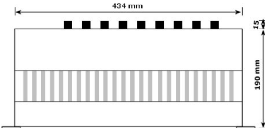
Vista Superior
